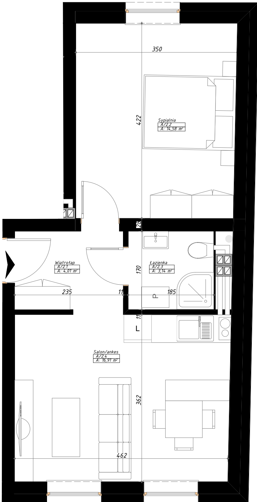
UKŁAD FUNKCJONALNY MIESZKANIA A/2 (SKALA 1:50)
